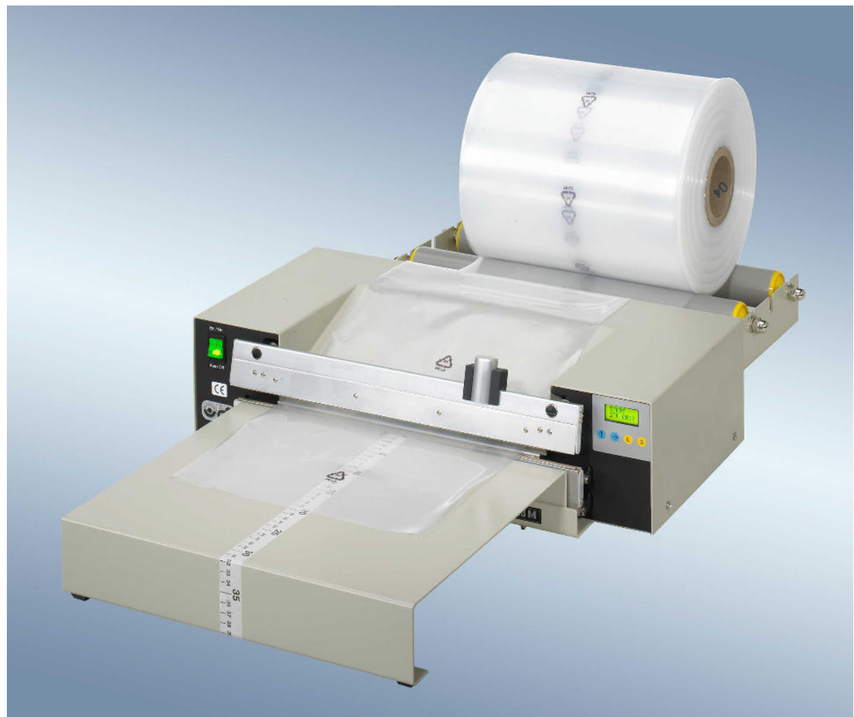
polystar® 413 M mit Schneidvorrichtung, Anstecktisch und Folienabroller
